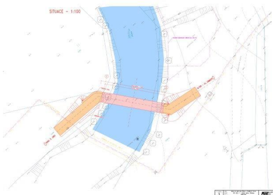
Obrázek 16 – Lávka Vícov – stavební záměr
