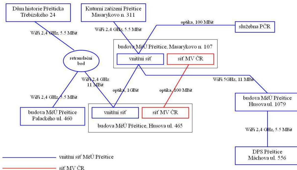
Schéma propojení budov MěÚ Přeštice
